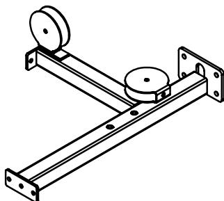
PART B-FRAME B, 1PCS.
